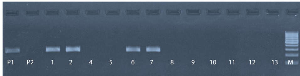
Рис. 1. Электрофоретический профиль маркерных фрагментов гена Rpf1 у гибридных сеянцев земляники (комбинация скрещивания Былинная × Фейерверк). P1 – Былинная, P2 – Фейерверк, 1–13 – гибридные сеянцы
