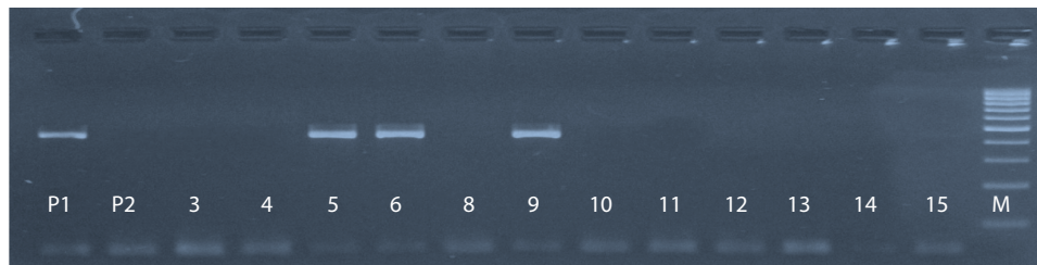
Рис. 2. Электрофоретический профиль маркерных фрагментов локуса 08 To-f у гибридных сеянцев земляники (комбинация скрещивания Былинная × Олимпийская надежда). P1 – Былинная, P2 – Олимпийская надежда, 3–15 – гибридные сеянцы
