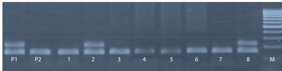
Рис. 3. Электрофоретический профиль маркерных фрагментов гена Rca2 у гибридных сеянцев земляники (комбинация скрещивания Malwina × Tea). P1 – Malwina, P2 – Tea, 1–8 – гибридные сеянцы
